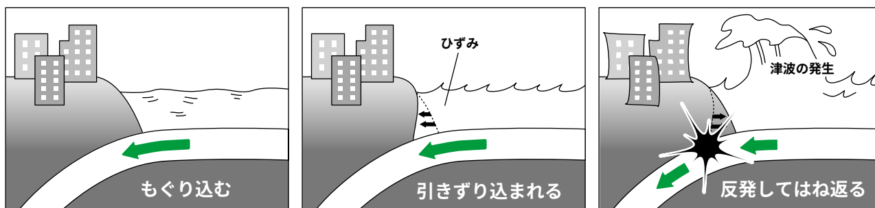
図2. 地震発生メカニズム
