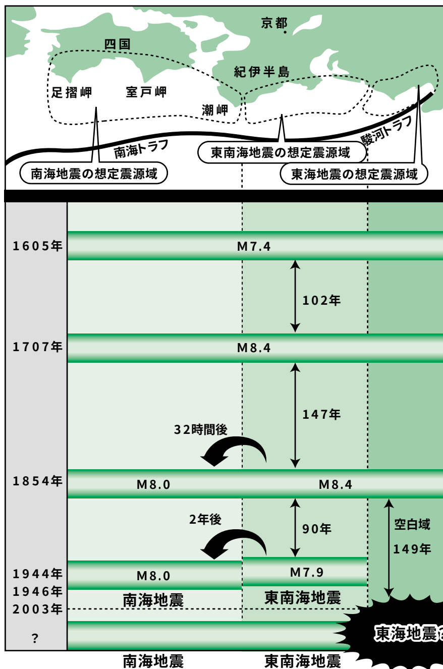
図1. 100～150年間隔で起こっている東海・東南海・南海地震
